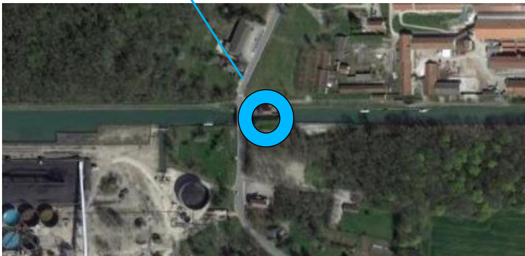
Ecluse 70 de Belvoye sur la Commune de Damparis Création d'un ponton d'attente pour la plaisance, plateforme bétonnée soutenue par des palplanches - PK 10.4 - coût d'investissement 25 000 € TTC
